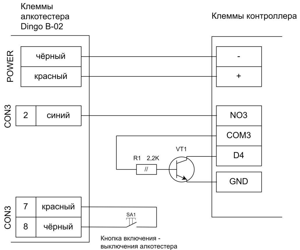
Подключение Динго В-02 к турникету.
