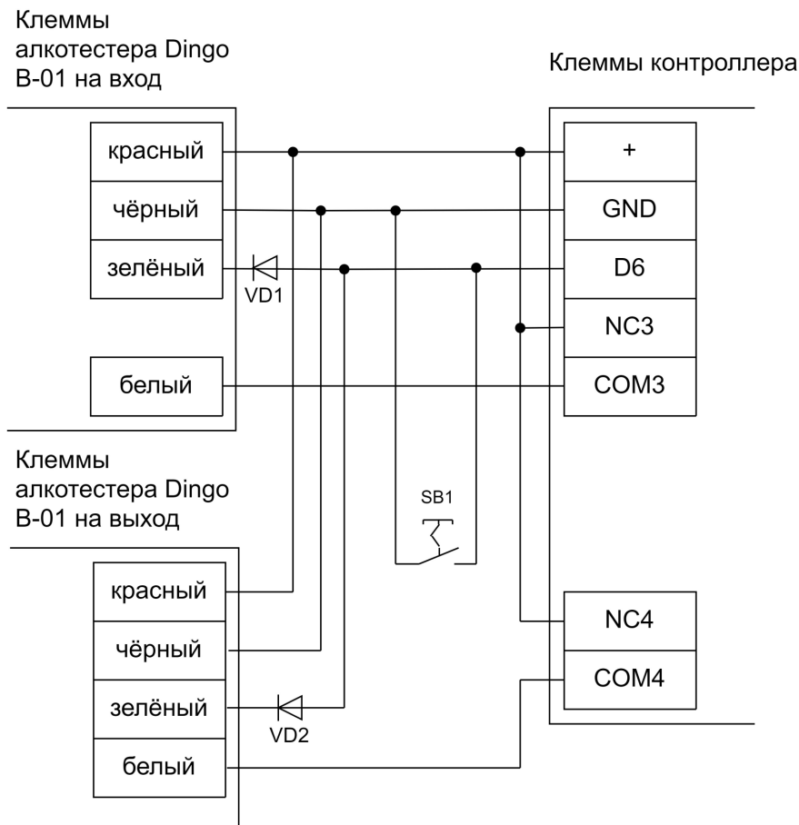
Подключение двух алкотестеров Динго B-01 к турникету.
