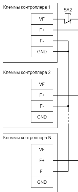
Подключение кнопки разблокирования к нескольким контроллерам.
